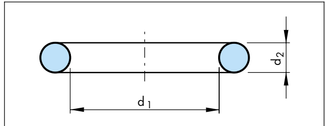
Figura 35 Dimensiones de una junta tórica
